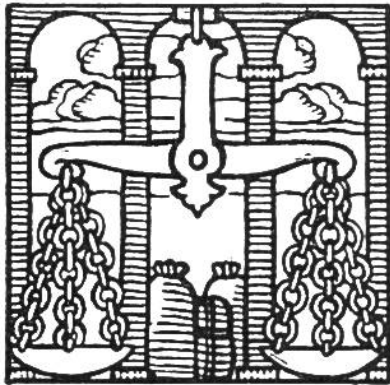
Sternbild Waage
