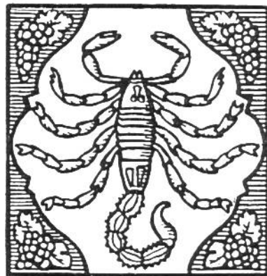
Sternbild Skorpion
