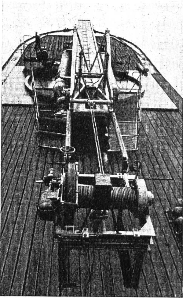
Die Schleudermaschine. Das aufragende Gestänge in der Mitte ist der Schlitten, auf den das Flugzeug aufgesetzt wird. Der Schlitten läuft auf 2 Schienen.
