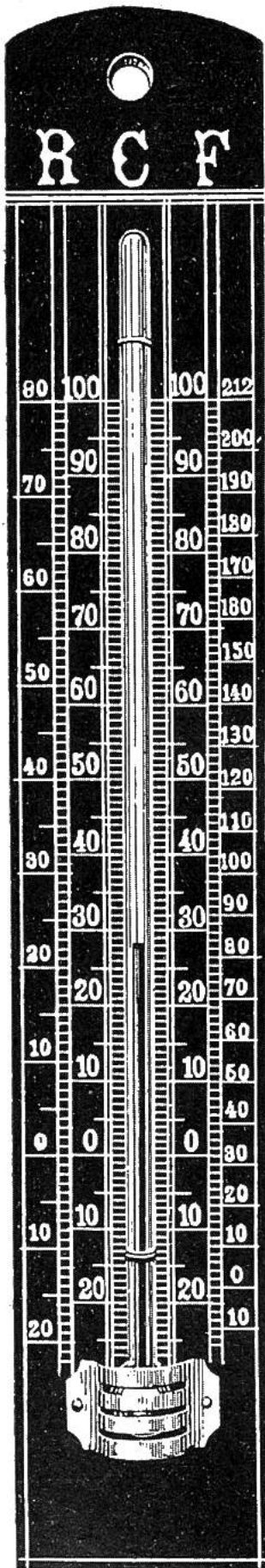
Réaumur-Celsius-Fahrenheit
