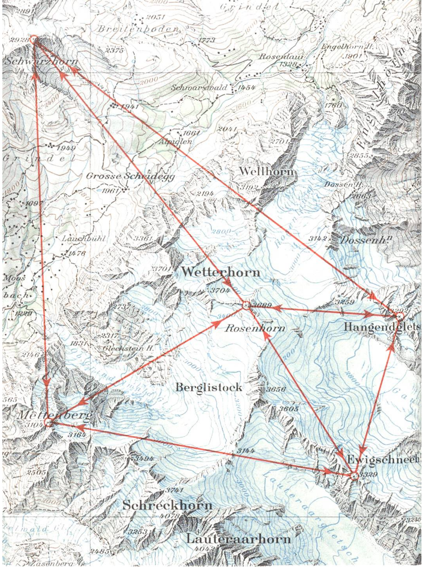
Teil eines Triangulationsnetzes III. Ordnung (Unterlage Landkarte 1:100 000).
