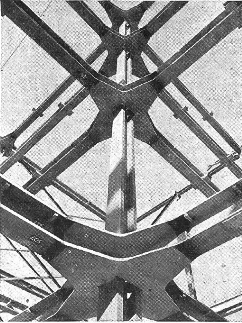
Warenhaus Jelmoli in Zürich-Oerlikon. Aus mächtigen Stahlprofilen ist eine Stütze zusammengeschnitten worden, bei welcher die Deckenunterzüge sternförmig zusammenkommen.
