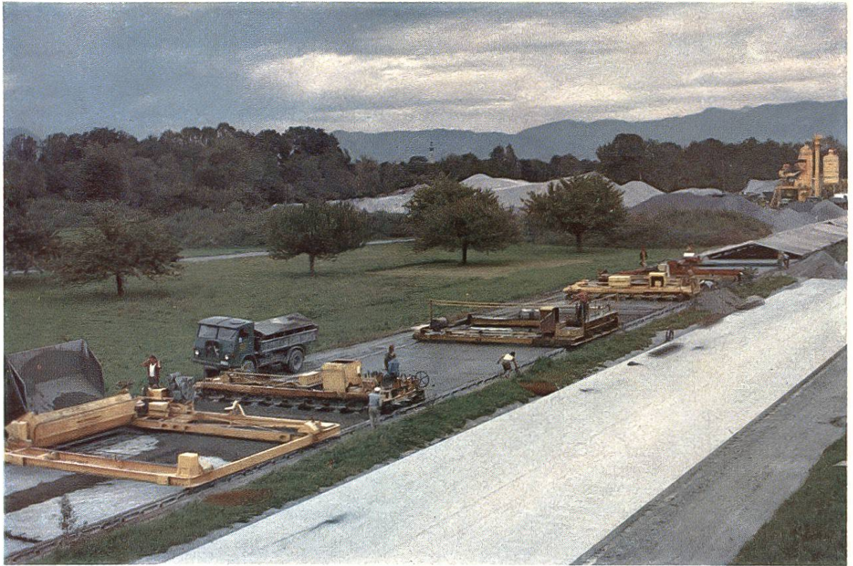
Betonbelagsbau der Nationalstrasse «N 1» bei St. Margrethen.
