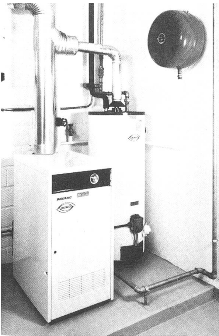
Moderner Gasheizkessel mit Heisswasserboiler im Privatwohnhaus.
