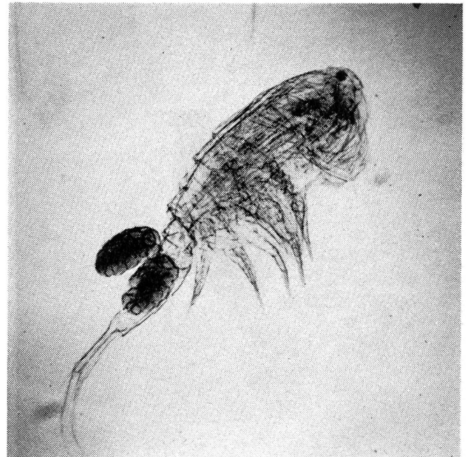
Abb. 3. Cyclops strenuus ♀
