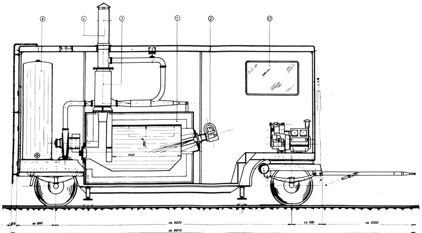
Abb. 1. Fahrbarer Tierkadaververbrennungs-ofen.
