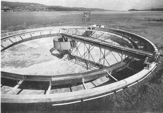
Kläranlage Horgen
