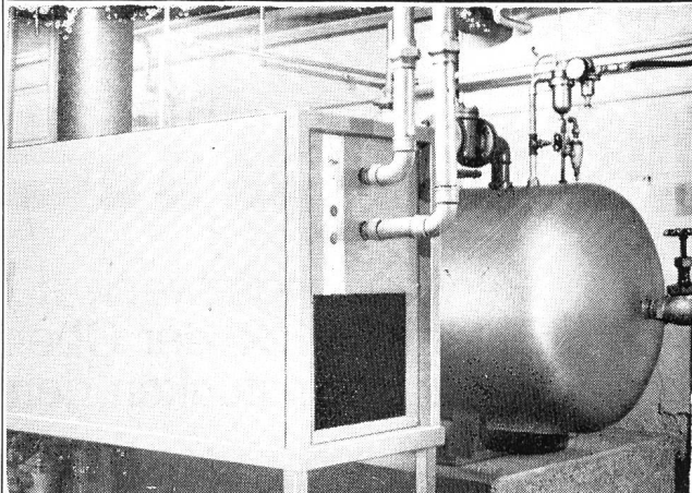
Druckluft-Trockner in Aerosol-Abfüllstation
