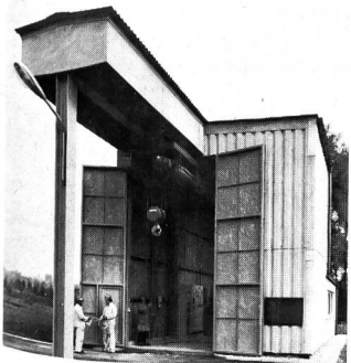
Gesamtansicht des oberirdischen Teils der Anlage Geiselbullach bei München mit Steuer- und Strahlenüberwachungsgeräten sowie Klärschlammbehälter
