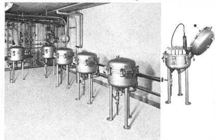
Ausschnitt aus einer Gruppe von 11 Entkeimungfiltern MF 31, Mineralquelle Eglisau, Leistung: 1000 l/min.
