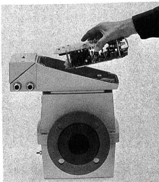
Abb. 2. Induktiver Durchflussmesser in neuer Kompaktbauweise mit angebautem Messumformer.
