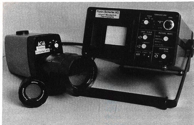
Abb. 5. Die Messausrüstung, bestehend aus Aufnahmeinheit und Monitor.
