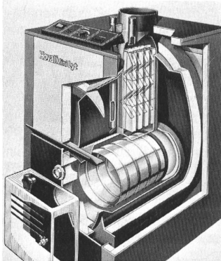
Schnittbild des Niedertemperaturkleinkessels Hoval MiniLyt.
