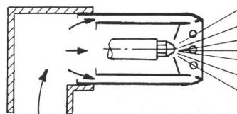
Warmluft-Spezialmischkopf.
