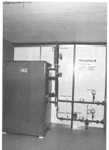
Beispiel einer Hausstation: rechts die Fernwärmeübergabestation, links die kompakte ausgebildete Hauszentrale, die gleichzeitig Raumwärme und Brauchwarmwasser liefert.
