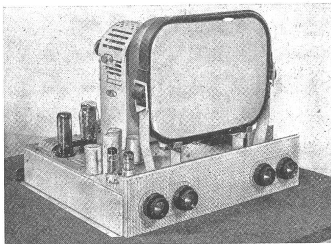
Das Chassis des Lorenz-Empfängers „Weltspiegel“ mit der metallbelagten Rechteck-Bildröhre eigener Konstruktion
