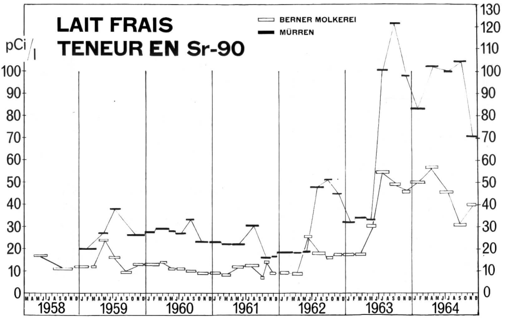
Fig. 8. Spezielle Strontium-90-Aktivität von Frischmilch aus dem Flachland (Bern 540 m) und aus einer Höhenlage (Mürren 1650 m). et de montagne (Mürren 1650 m). Frischmilch, Flachland. Lait frais, plaine. Frischmilch, Höhenlage. Lait frais, montagne.
