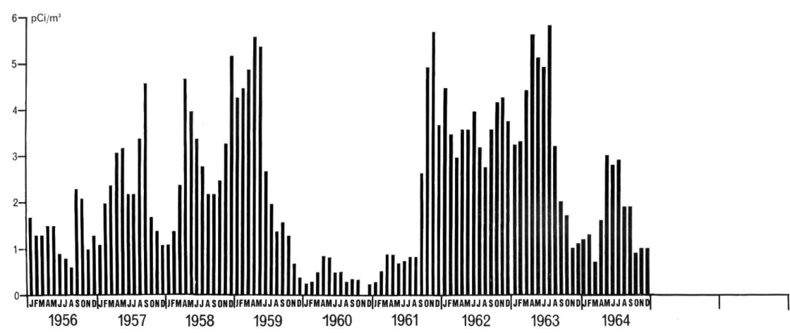
Fig. 2. Monatliche Mittelwerte der spezifischen Gesamt-Betaaktivität der Luft, bezogen auf 760 mm Hg und 0° C, für die Messstelle Payerne von 1956 bis 1964. Fig. 2. Moyennes mensuelles de l'activité spécifique bêta totale de l'air, à 760 mm Hg et 0° C mesurées à la station de Payerne de 1956 à 1964.
