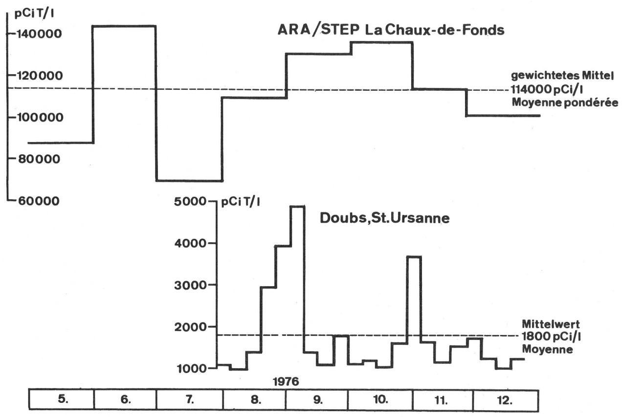
Fig. 14 Tritium im Wasser der ARA von La Chaux-de-Fonds und im Doubs Tritium dans l'eau de la STEP de La Chaux-de-Fonds et dans le Doubs (EAWAG, LFR)
