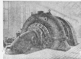
Turbine de 22,750 chx.
