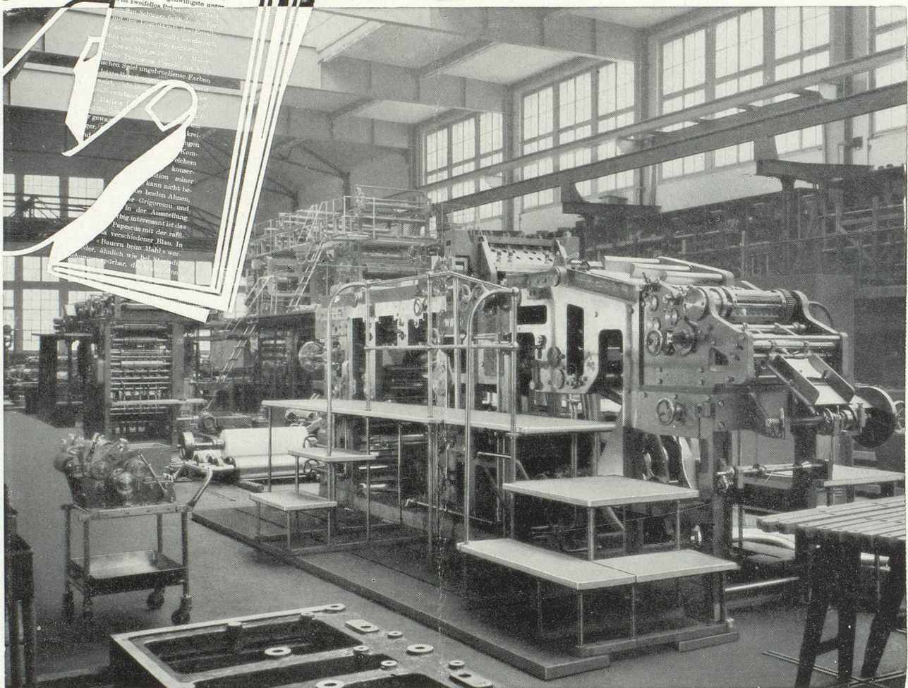
Vue partielle des halles de montage des rotatives WIFAG
