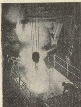
Notre couverture : Coulée. Vue prise dans une fonderie d'acier de Georges Fischer, Société anonyme à Schaffhouse (Suisse)
