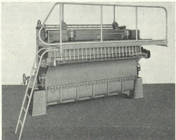
Caisse d'arrivée de pâte à réglage précis.
