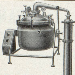
Appareil à distiller sous vide, électrique. Inoxydable et basculable, chauffage par rayonnement, régulation automatique jusqu'à 350° C.
