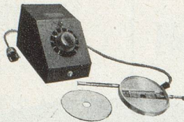
Platine chauffante électrique pour microbactériologie. Adaptable sur tous les microscopes, en particulier pour la bactériologie et parasitologie et pour d'autres emplois. Régulée jusqu'à 65° C.
