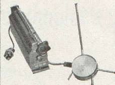
Appareil pour la microdétermination du point de fusion. Adaptable sur tous les microscopes. a) Avec thermo-élément et instrument de lecture de précision. b) Avec thermomètre à mercure. Utilisable entre 0 et 400° C.
