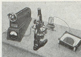
Appareil pour la microdétermination du point de fusion. Adaptable sur tous les microscopes. a) Avec thermo-élément et instrument de lecture de précision. b) Avec thermomètre à mercure. Utilisable entre 0 et 400° C.
