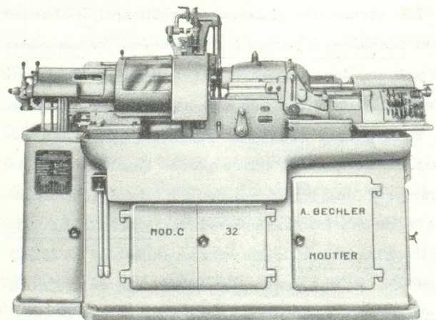
Tour automatique à décolleter à poupée mobile.
