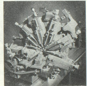
Les 6 outils radiaux d'un tour à décolleter.
