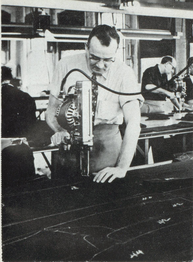
Machine à couper les tissus.
