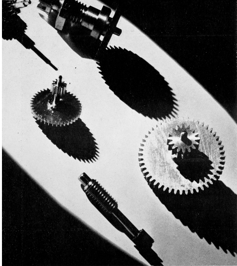
Ci-dessus : pièces de décolletage. A droite: il faudrait 4 800 000 de ces billes pour remplir une bouteille d'un litre! Quelques-unes d'entre elles sont ici photographées sur un disque de phon. Ces billes minuscules (diamètre : 65/100 de millimètre) composent le roulement d'une montre automatique. Page de droite : dans un bureau d'études à Ébauches S.A.
