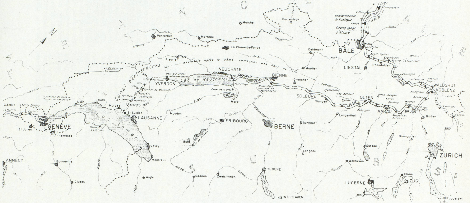
Extrait du plan n° 12.645 (janvier 1961) du Service fédéral des Eaux, Berne Projet du tracé du canal du Rhône au Rhin en Suisse
