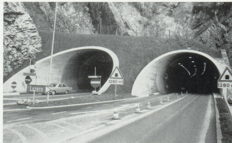
Entrée sud du tunnel du Lopper autoroute près de Lucerne.
