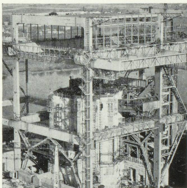
La centrale nucléaire St. Laurent de l'Electricité de France, d'une puissance de 480 000 kW, est équipée de générateurs de vapeur, d'un système de réglage et de soufflantes de CO 2 Sulzer.
