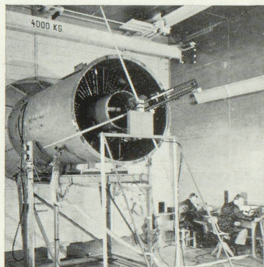
Installation d'essais dans le tunnel aérodynamique pour l'étude du comportement aux vibrations de faisceaux tubulaires «Helix» destinés aux générateurs de vapeur Sulzer pour réacteurs à hautes températures.
