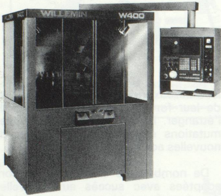
W-400 Centre d'usinage 5 axes, broche inclinable, magasin à 12, 24, 36 ou 48 outils, commande numérique NUM ou General Electric
