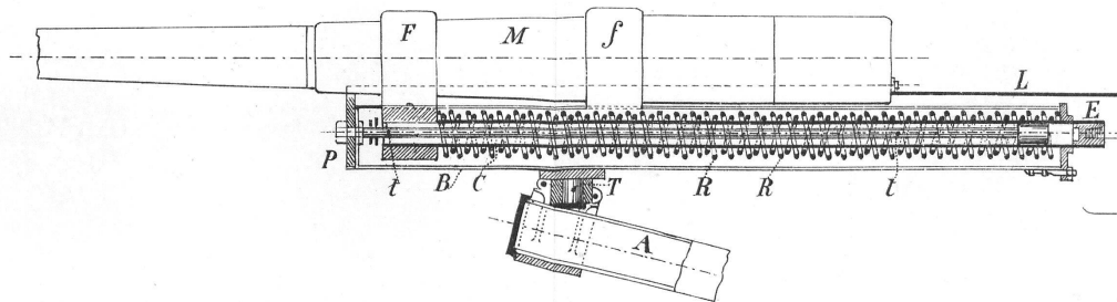
fig. 1. Bouche à feu et berceau.
