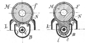
fig. 3 Coupe suivant f fig. 2 Coupe suivant F.
