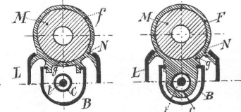
fig. 3 Coupe suivant f fig. 2 Coupe suivant F.
