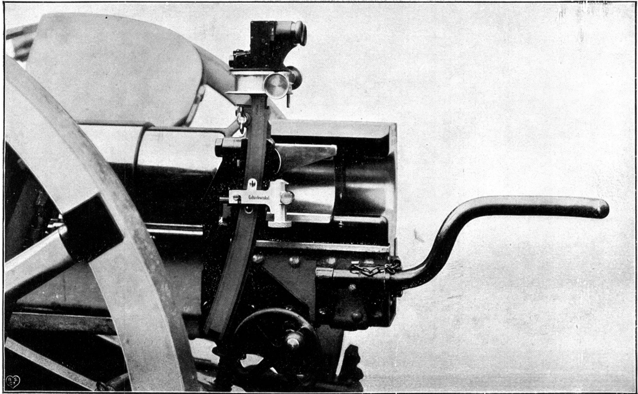
Fig. 18. Hausse Krupp à lunette pour canon à recul sur l'affût. Vue latérale.
