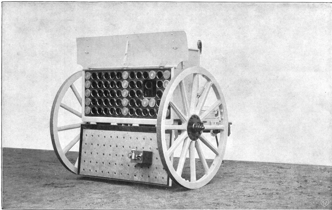
Arrière-train de caisson non renversable.
