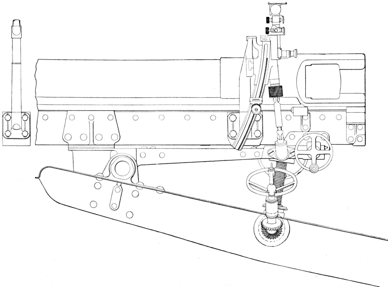
Appareil de mire. Vue de profil.
