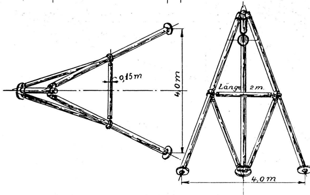
FIG. 20. Plan
