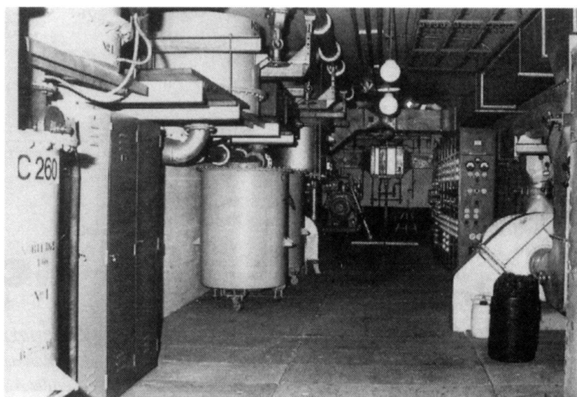
La salle des machines du Helderberg: indispensable à la survie à long terme des hommes.
