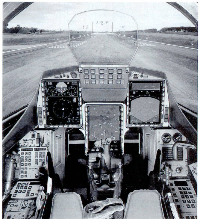
Le « bureau » du JAS-39 Gripen C/D . Toutes les illustrations: Gripen International.
