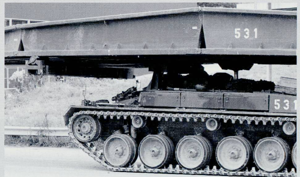
Le char poseur de ponts 68/88 permet les franchissements jusqu'à 18 mètres d'engins jusqu'à 60 tonnes.
