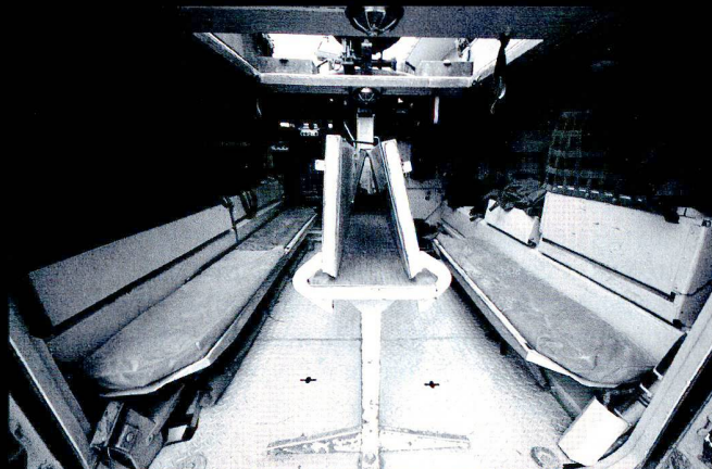
Char de commandement 63, avec une table escamotable.
