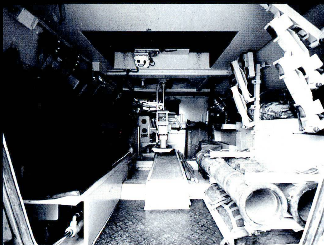
Compartment de combat du chasseur de chars TOW- Piranha .
