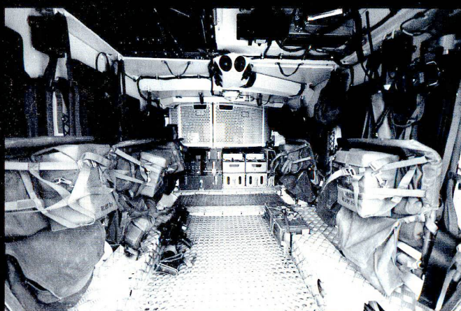
Intérieur du char de grenadiers 2000, prêt au combat.
