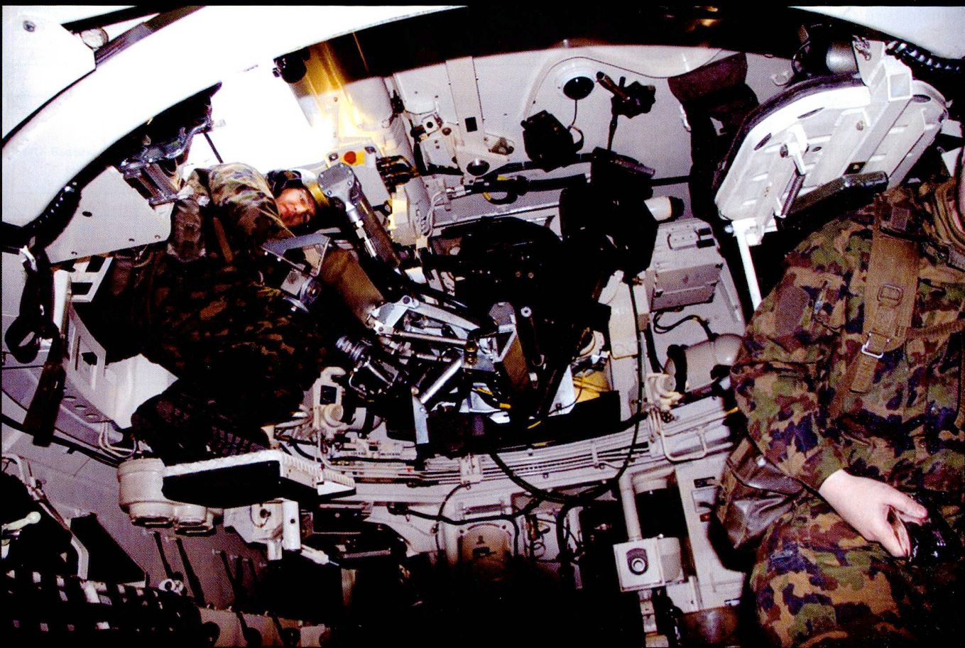
Compartiment de combat de l'obusier blindé M-109.
