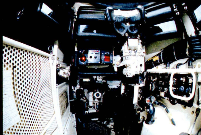
Poste de combat (pointeur/commandant) du char Léo .
