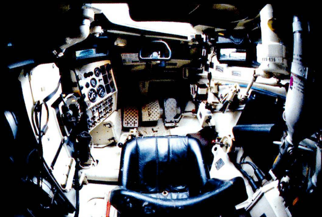
Poste du pilote du char 87 Léopard .
