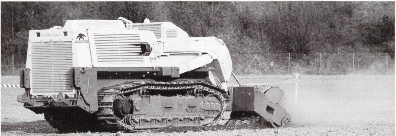
Machine de déminage DIGGER D-250 en pleine action.
