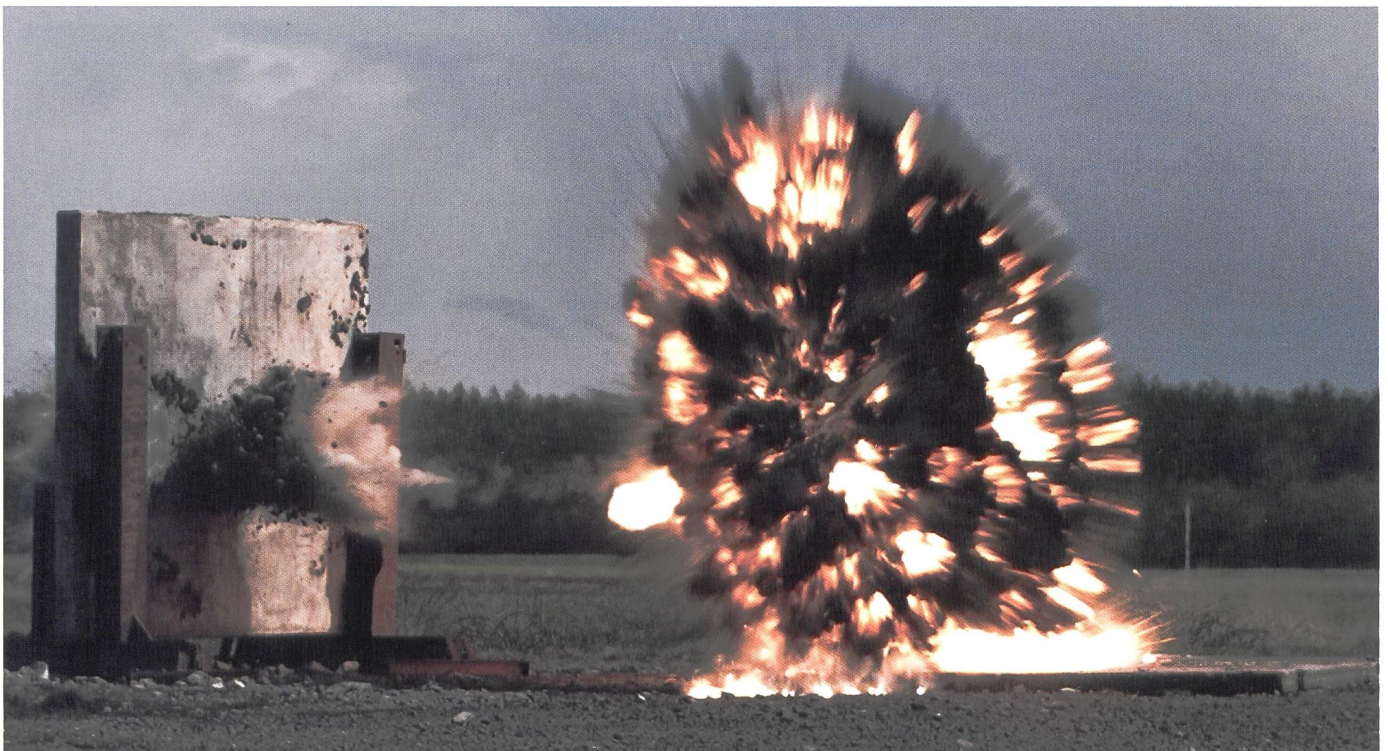
Perforation d'un mur avec détonation successive d'un obus explosif 15.5 cm DM121 de Rheinmetall. Photo © Rheinmetall Waffe Munition GmbH.
