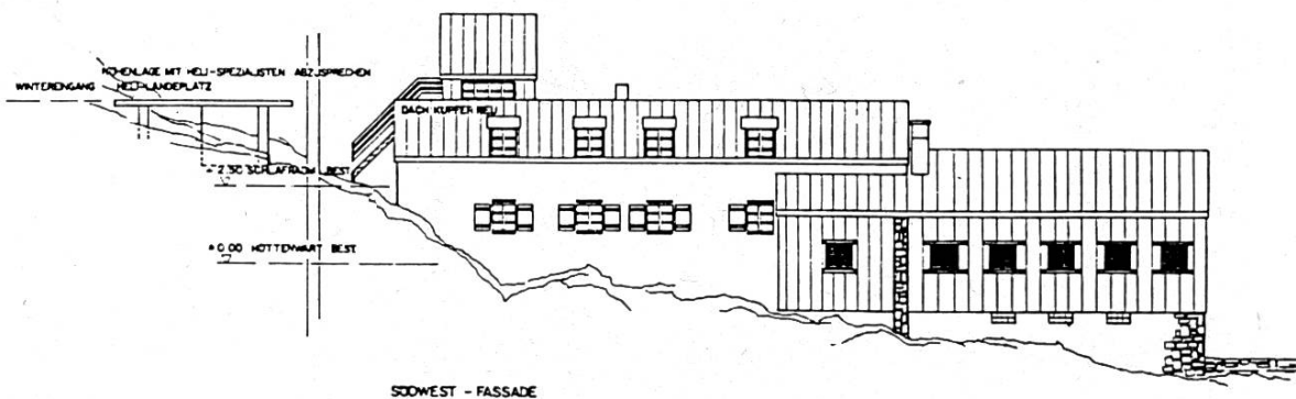
SOWEST – FASSADE
