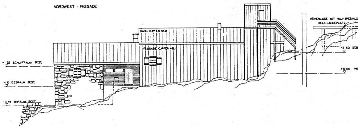
NOROOST – FASSADE
