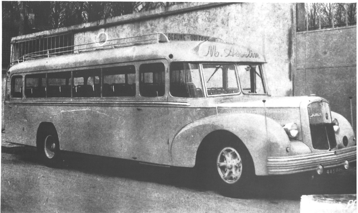
Bild unten: Saurer 3C Motor CT 3 D, Baujahr 1953, Carrosserie von Peperl in Rennes. 34 Sitzplätze.
