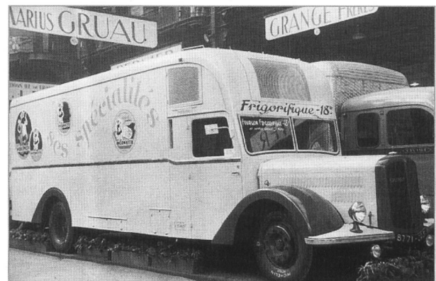
Kühlauflieger von David auf 3CT1D. Das Kühlaggregat ist oberhalb des Fahrerhauses in den Aufbau integriert
