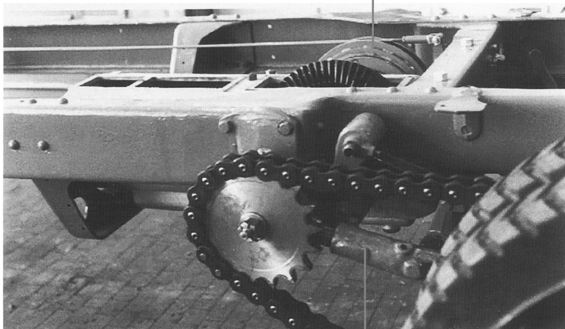
Antriebskettenrad mit 18 Zähnen
