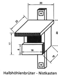
Halbhöhlenbrüter - Nistkasten
