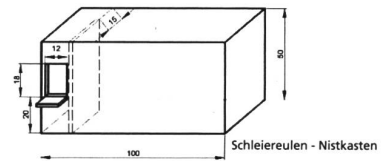
Schleiereulen - Nistkasten
