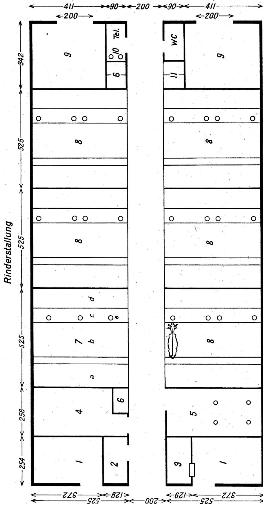
Abb. 2 Ganzer Komplex mit Mauern und Zwischenwänden: 25,70 × 13,20 m. 1. Absonderungsstall für 2 Großtiere; 2. Stallgeräte; 3. Instrumente, Medikamente; 4. Milehzimmer; 5. Untersuchungsraum mit Notstand; 6. Heu- und Strohabwurf; 7. Abteilung für 3 Tiere; 8. Abteilung für 4 Tiere; 9. Abkalbeboxe; 10. Kraffutter-Auslaufrohre; 11. Aufgang zur Heubühne.
