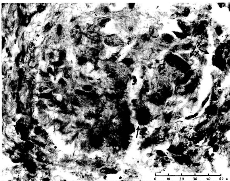
Abb. 6 Giraffe, Jejunallmkn. v. Gieson, Vergrößerung etwa 500 \times . Epitheloid- und Riesenzell-Granulom. Vor den Pfeilen: Gruppen von m. o. w. katabiotischen Kernen von Riesenzellen.
