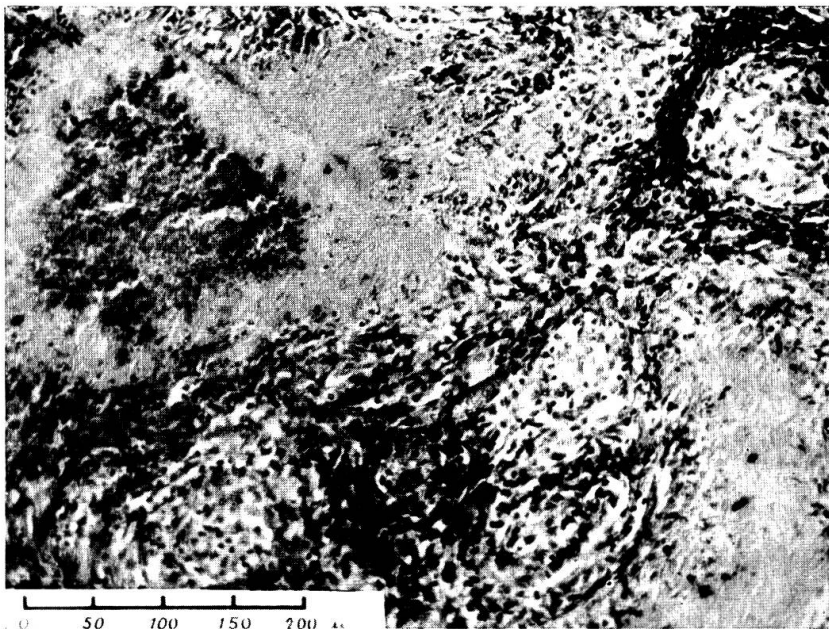
Abb. 5 Vierhorn-Antilope. Ausschnitt aus einem kleinen Lungentuberkulom. v. Gieson, Vergrößerung etwa 300 \times . Links oben und rechts unten Nekroseherdchen mit Verkalkungen. Dazwischen lockere zellige Knötchen, rechts oben mit Epitheloiden.
