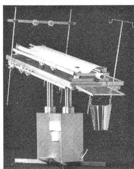
OP-Tisch: Hub und Neigung elektrisch über Fusstasten, Versorgungsschienen
